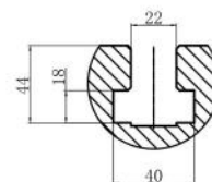
T形槽尺寸
